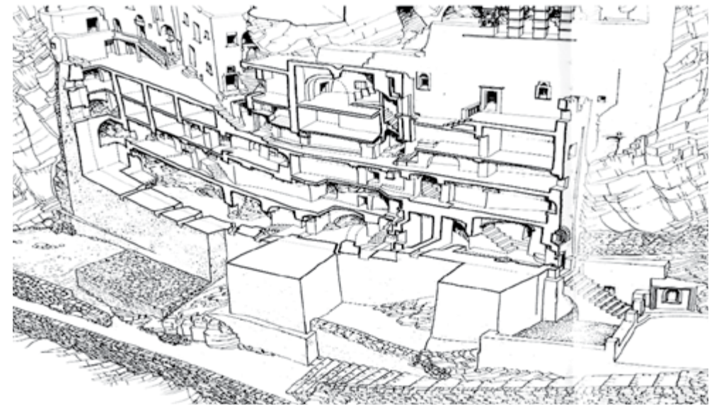
Αξονομετρική τομή του εσωτερικού της Μονής, (από το βιβλίο της Λίλας Μαραγκού «Η Μονή της Παναγίας της Χοζοβιώτισσας στην Αμοργό»)
